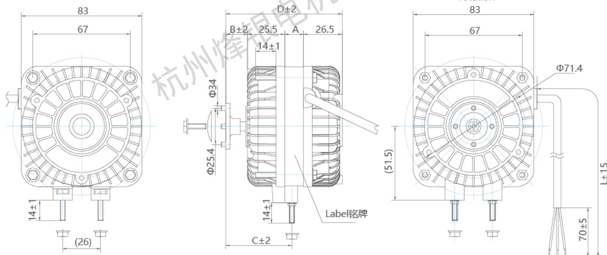
电机性能参数表 Motor performance parameter table
